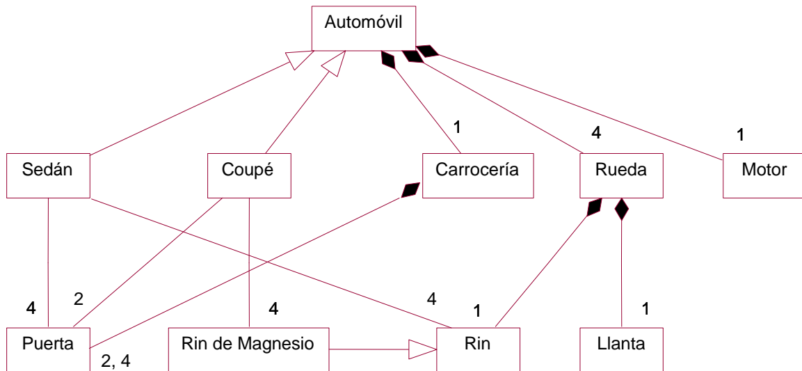
Figura 4.96. Diagrama de clases para un ensamblado describiendo un Automóvil que contiene varios componente: un Motor , una Carrocería , y cuatro Ruedas . Pueden haber diferentes tipos de Automóvil , Deportivo o Sedan , conteniendo Rin de Magnesio o una Parrilla para Maletas , respectivamente. Rin de Magnesio es subclase de Rin , el cual es componente de Rueda al igual que Llanta .
