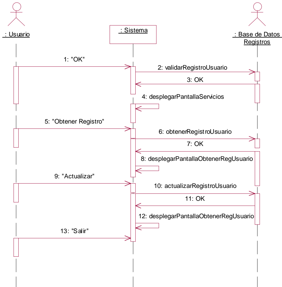
Figura 10.7 Diagrama de secuencias para Actualizar Registro Usuario del caso de uso Registrar Usuario .
