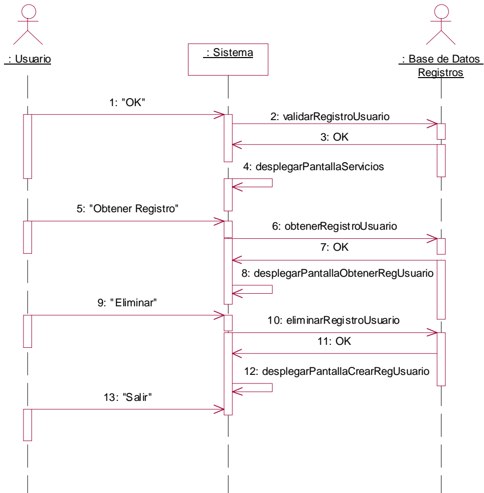
Figura 10.12 Diagrama de secuencias Eliminar Registro Usuario del caso de uso Registrar Usuario .
