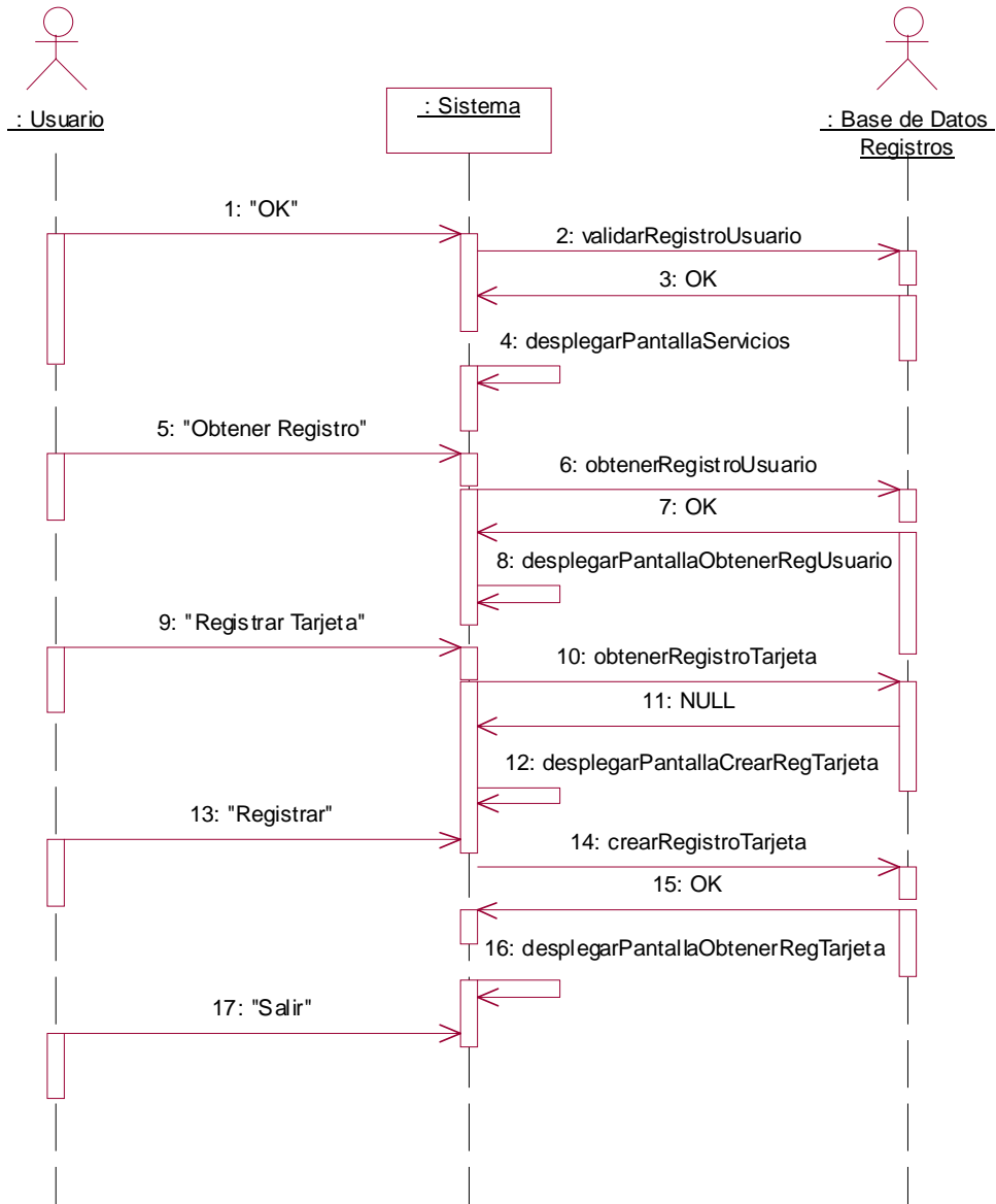
Figura 10.16 Diagrama de secuencias Crear Registro Tarjeta del caso de uso Registrar Tarjeta .
