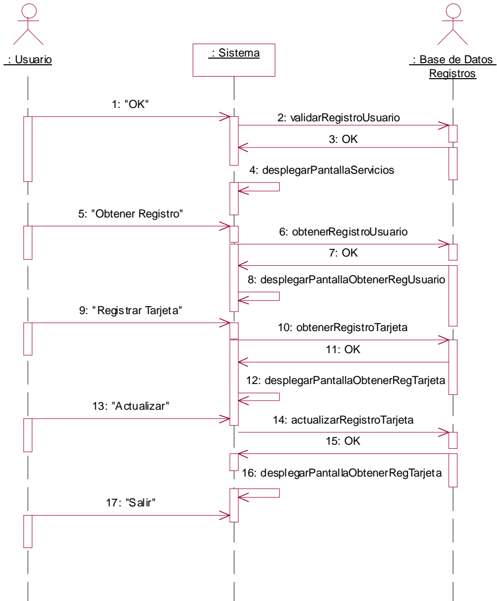
Figura 10.21 Diagrama de secuencias Actualizar Registro Tarjeta del caso de uso Registrar Tarjeta .
