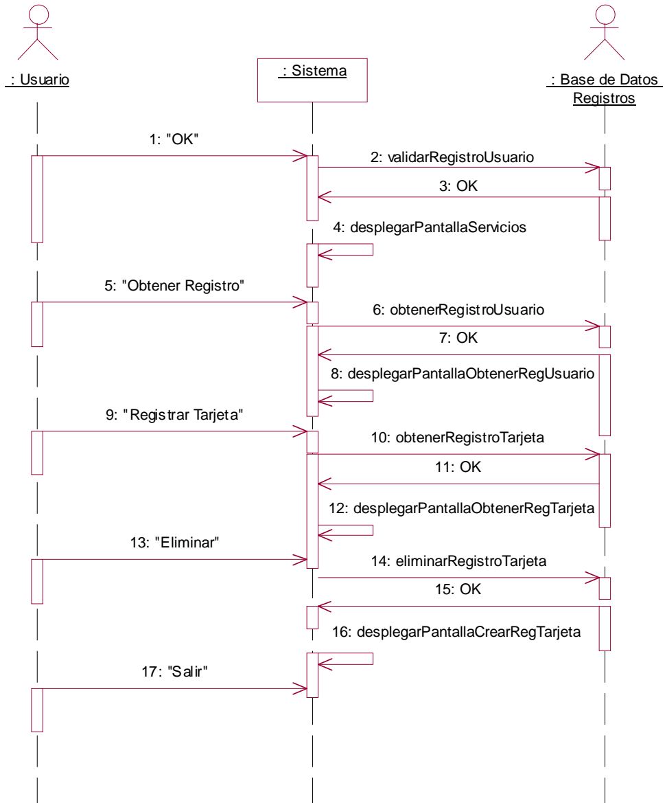
Figura 10.24 Diagrama de secuencias Eliminar Registro Tarjeta del caso de uso Registrar Tarjeta .
