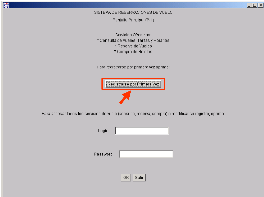
Figura 2 La secuencia Crear Registro Usuario comienza con el usuario oprimiendo el botón “Registrarse por Primera Vez” en la PantallaPrincipal (P-1).
