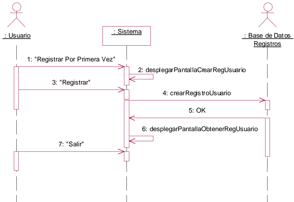
Figura 1 Diagrama de secuencia Crear Registro Usuario del caso de uso Registrar Usuario .
